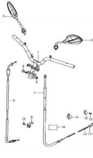
Fig.36 GUIDAO (T06-S330-0035) REF.No.
