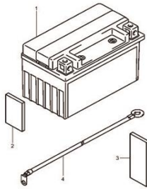
Fig.21 BATERIA (T06-S190-0007) REF.No.
