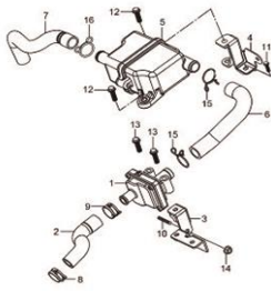
Fig.14 BOMBA DE OLEO (T06-S130-0007) REF.No.
