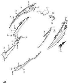
Fig.34 TAMPA DO CHASSI (T06-S310-0022) REF.No.
