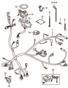
Fig.27 CHICOTE (T06-S250-0032) REF.No.
