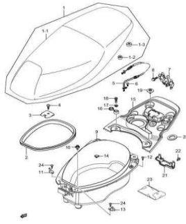
Fig.41 ASSENTO (T06-S380-0016) REF.No.
