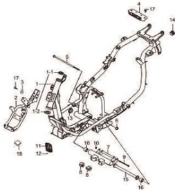
Fig.28 CHASSI (T06-S260-0056) REF.No.
