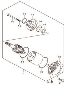
Fig.19 MOTOR DE PARTIDA (T06-S170-0003) REF.No.
