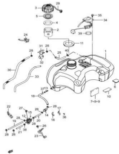
Fig.32 TANQUE DE COMBUSTIVEL (T06-S290-0014) REF.No.
