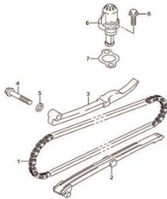
Fig.8 CORRENTE DE COMANDO (T06-S080-0004) REF.No.
