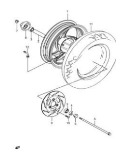
Fig.43 RODA DIANTEIRA (T06-S410-0010) REF.No.
