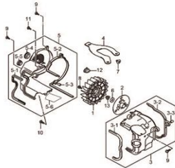
Fig.15 VENTOINHA (T06-S135-0005) REF.No.
