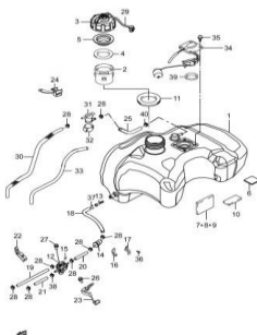
Fig.32 TANQUE DE COMBUSTIVEL (T06-S290-0014) REF.No.
