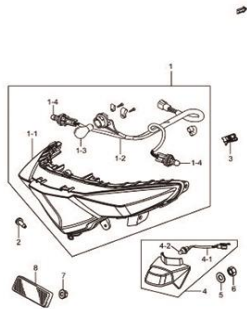
Fig.26 LANTERNA TRASEIRA (T06-S240-0008) REF.No.
