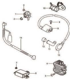
Fig.22 ELETRICA (T06-S200-0012) REF.No.
