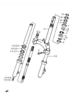
Fig.42 SUSPENSÃO DIANTEIRA (T06-S400-0008) REF.No.
