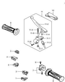
Fig.37 MANETE E MANOPLAS (T06-S340-0016) REF.No.
