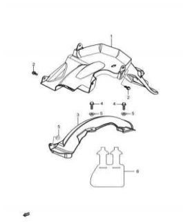
Fig.39 CARENAGEM DO GUIDAO (T06-S365-0010) REF.No.
