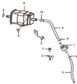
Fig.11 FILTRO DE AR (T06-S100-0013) REF.No.
