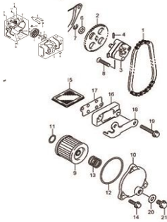
Fig.14 BOMBA DE OLEO (T06-S130-0007) REF.No.
