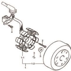
Fig.20 MAGNETO (T06-S180-0004) REF.No.
