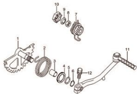
Fig.18 PEDAL DE PARTIDA (T06-S165-0001) REF.No.
