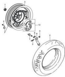
Fig.48 RODA TRASEIRA (T06-S460-0011) REF.No.
