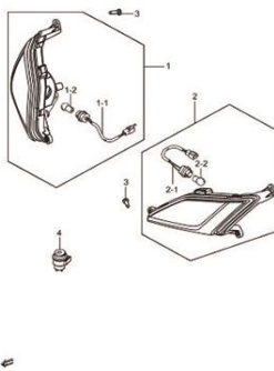
Fig.26 LANTERNA TRASEIRA (T06-S240-0008) REF.No.
